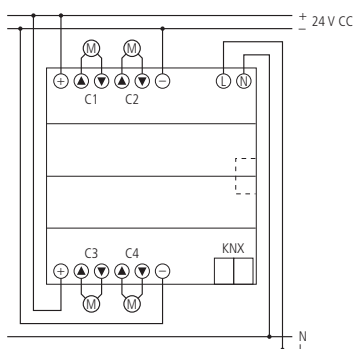
JMG 4 24V CC KNX
