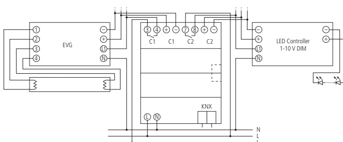
SMG 2 S KNX
