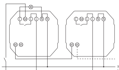
SPHINX 104-360 AP, SPHINX 104-360
