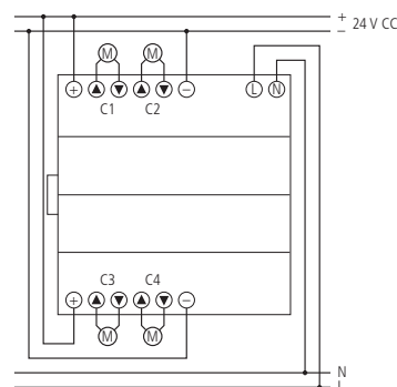
JME 4 24V CC KNX
